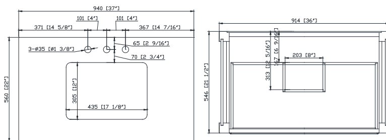
Top / Cima
