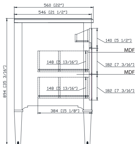
Side / Lado
