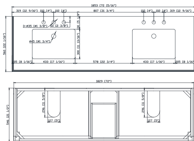
Top / Cima
