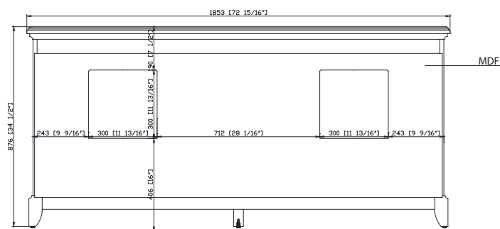
Back / Atrás
