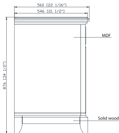
Side / Lado
