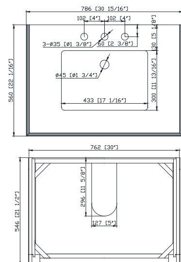
Top / Cima
