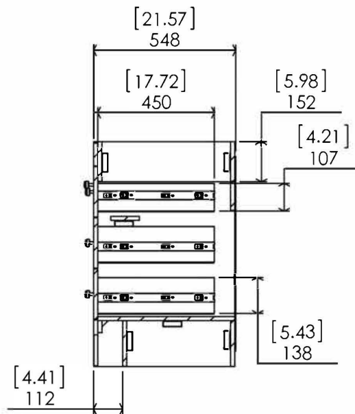
SECTION A-A
