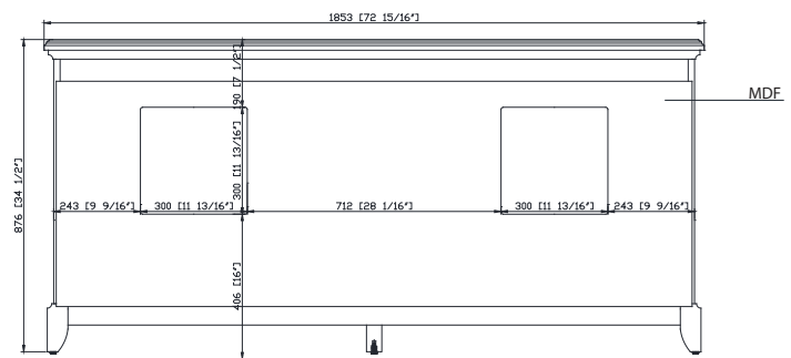
Back / Atrás
