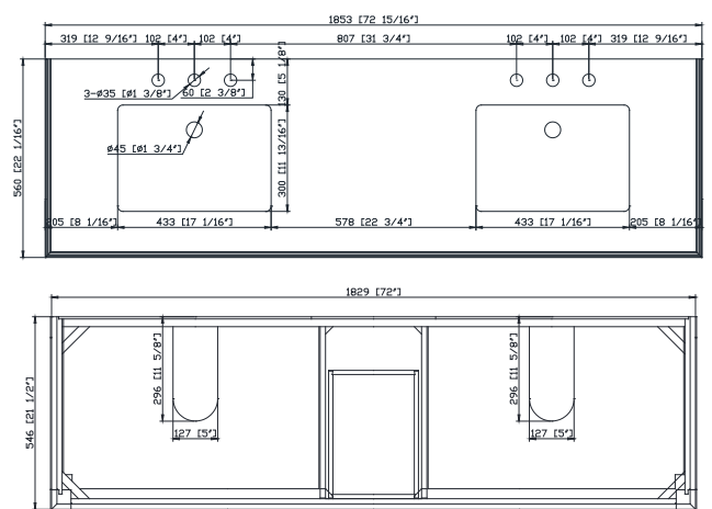
Top / Cima
