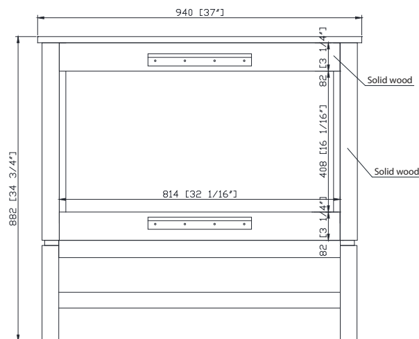
Back / Atrás
