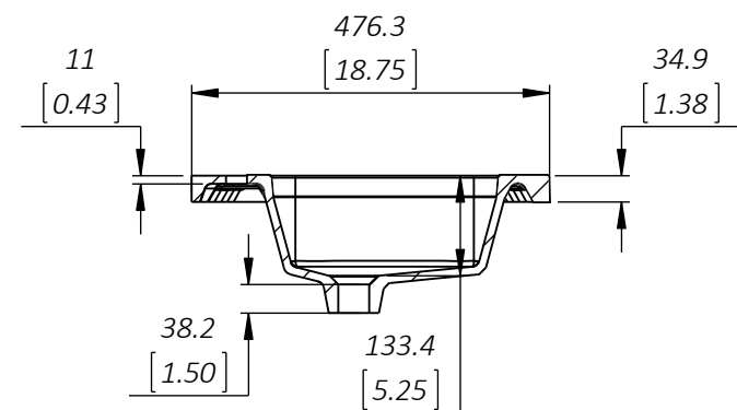
SECTION T-T SCALE 1 : 11
