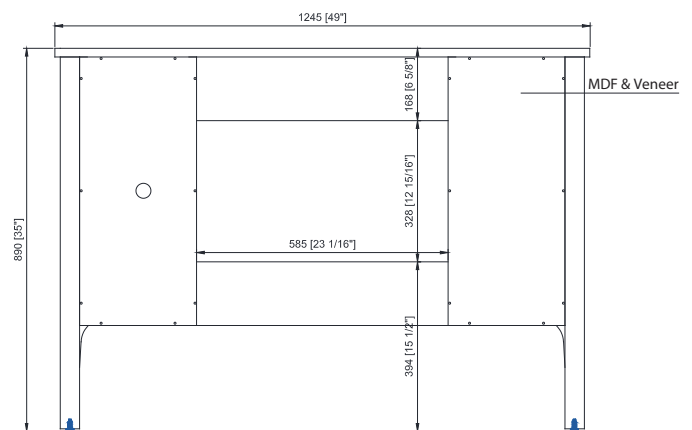
Back / Atrás
