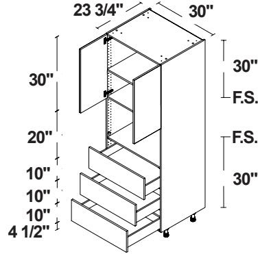
MICROONDAS 1 2 PUERTAS / 3 CAJONES
