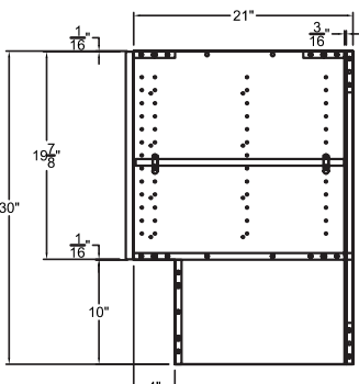
GABINETE DE TOCADOR ALTO ADA DE 30"
