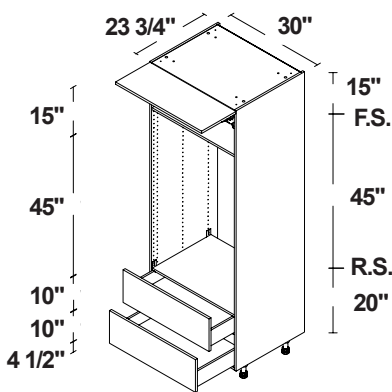
MICRO/HORNO DE PARED 2 1 PUERTA ELEVABLE / 2 CAJONES
