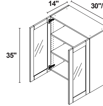
35" DE ALTURA/2 PUERTAS DE VIDRIO*
