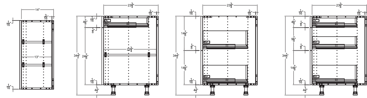
GABINETE DE PARED GABINETE BASE GABINETE BASE DE DOS CAJONES GABINETE BASE DE TRES CAJONES
