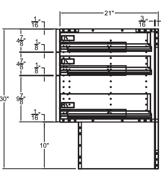
GABINETE DE TOCADOR ALTO CON TRES CAJONES ADA DE 30"
