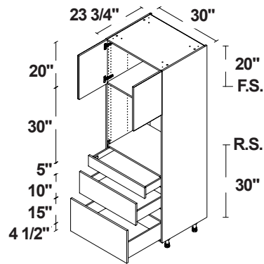
HORNO SIMPLE 4 2 PUERTAS / 3 CAJONES
