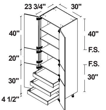
6 PUERTAS / 3 CAJONES INTERIORES
