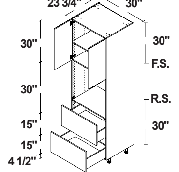
HORNO SIMPLE 3 2 PUERTAS / 2 CAJONES
