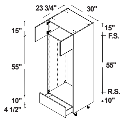
HORNO DOBLE 3 2 PUERTAS / 1 CAJÓN
