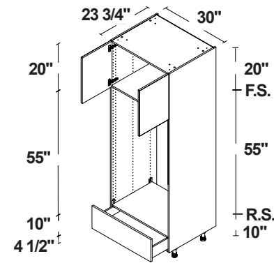
HORNO DOBLE 3 2 PUERTAS / 1 CAJÓN
