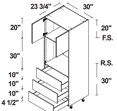
HORNO SIMPLE 4 2 PUERTAS / 3 CAJONES
