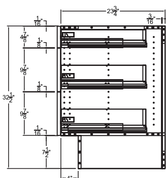
GABINETE BASE ALTO CON TRES CAJONES ADA DE 32 1/2"
