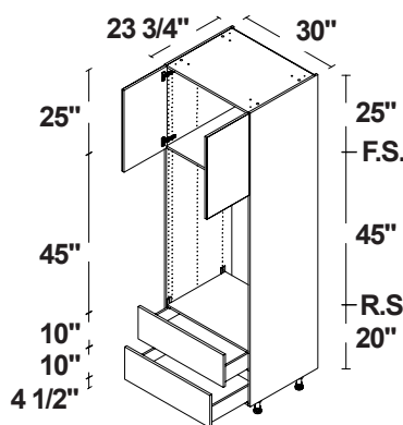
HORNO SIMPLE 3 2 PUERTAS / 2 CAJONES
