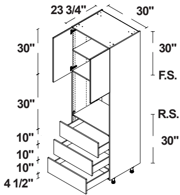
HORNO SIMPLE 3 2 PUERTAS / 3 CAJONES
