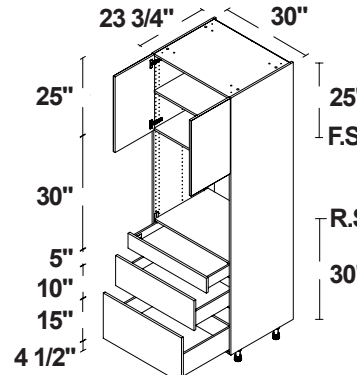
HORNO SIMPLE 3 2 PUERTAS / 3 CAJONES
