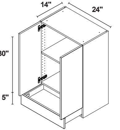
35" DE ALTURA/ 2 PUERTAS / 1 CAJÓN
