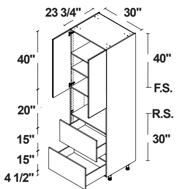
MICROONDAS 1 2 PUERTAS / 2 CAJONES
