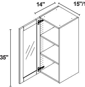
35" DE ALTURA/1 PUERTA DE VIDRIO*
