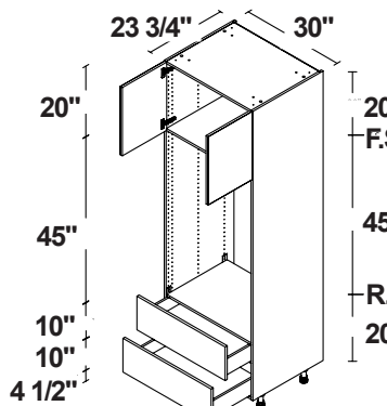
MICRO/HORNO DE PARED 2 2 PUERTAS / 2 CAJONES
