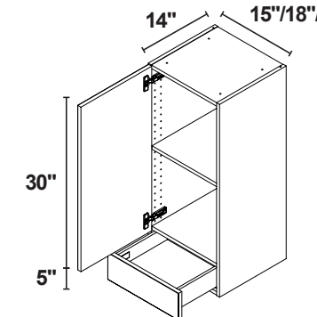
35" DE ALTURA/1 PUERTA/1 CAJÓN
