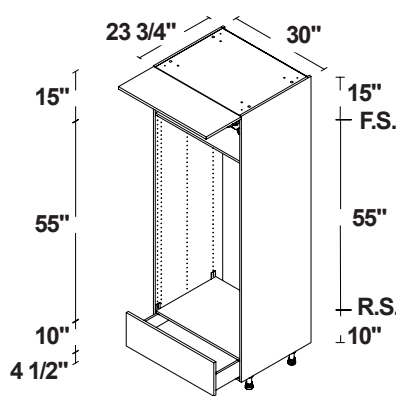
HORNO DOBLE 3 1 PUERTA ELEVABLE / 1 CAJÓN
