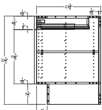
GABINETE BASE ALTO ADA DE 32 1/2"
