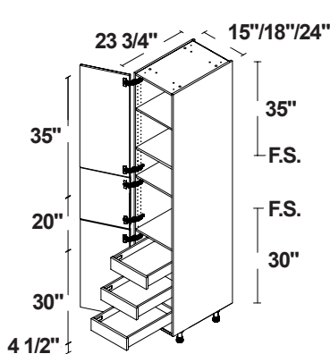
3 PUERTAS / 3 CAJONES INTERIORES
