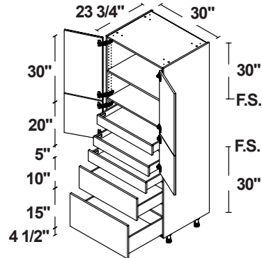
4 PUERTAS / 3 CAJONES / 2 CAJONES INTERIORES
