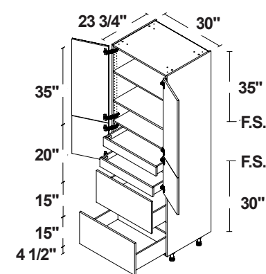
4 PUERTAS / 2 CAJONES / 2 CAJONES INTERIORES
