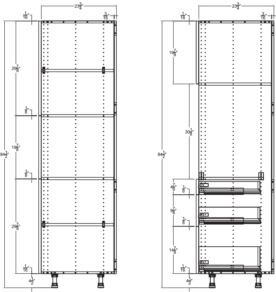
GABINETE PARA UTENSILIOS GABINETES ALTO PARA MICROONDAS 3D
