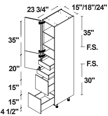
2 PUERTAS / 2 CAJONES / 2 CAJONES INTERIORES
