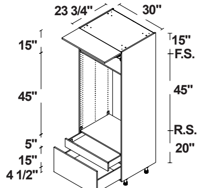
MICRO/HORNO DE PARED 2 1 PUERTA ELEVABLE/ 2 CAJONES
