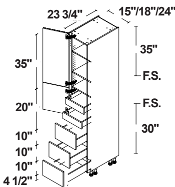
2 PUERTAS / 3 CAJONES / 2 CAJONES INTERIORES
