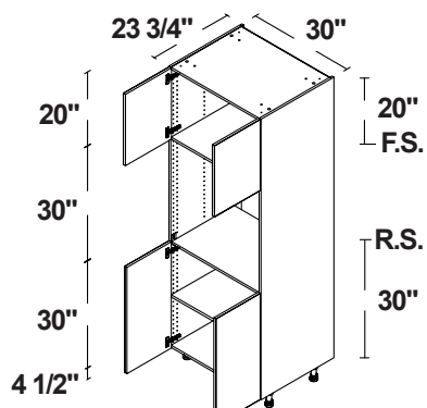
HORNO SIMPLE 4 / 4 PUERTAS
