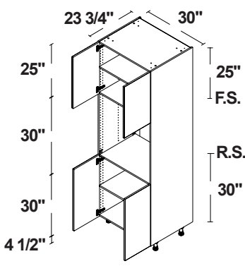
HORNO SIMPLE 3 4 PUERTAS
