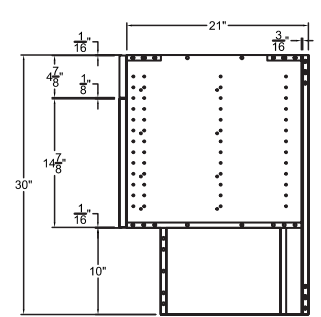
GABINETE DE TOCADOR ALTO ADA DE 30"
