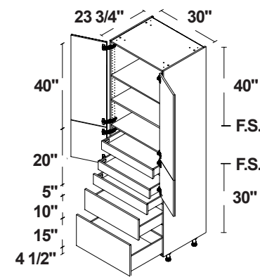
4 PUERTAS / 3 CAJONES 2 CAJONES INTERIORES
