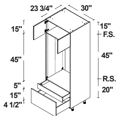
MICRO/HORNO DE PARED 2 2 PUERTAS / 2 CAJONES
