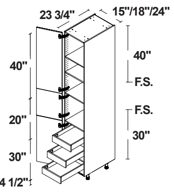
3 PUERTAS / 3 CAJONES INTERIORES
