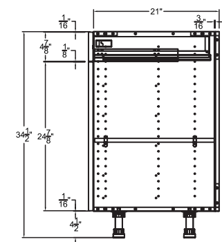
GABINETE DE TOCADOR DE ALTO ESTÁNDAR DE 34 1/2"
