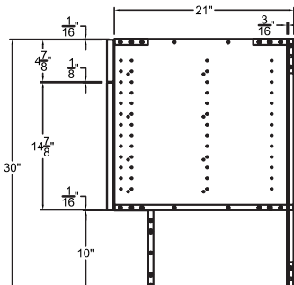
GABINETE DE TOCADOR ALTO ADA DE 30"
