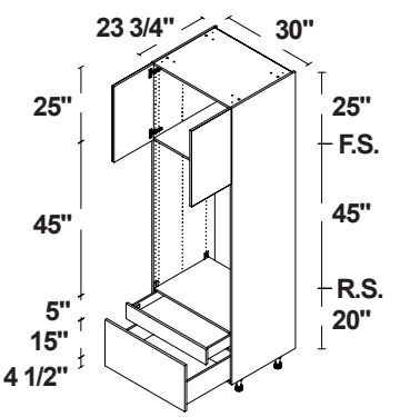
MICRO/HORNO DE PARED 2 2 PUERTAS / 2 CAJONES
