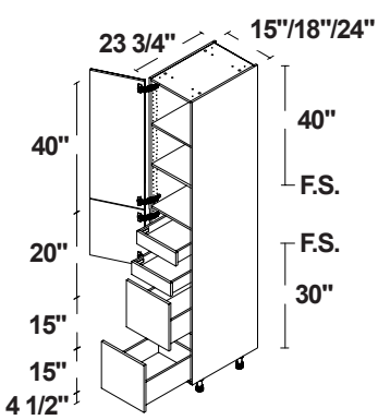
2 PUERTAS / 2 CAJONES / 2 CAJONES INTERIORES
