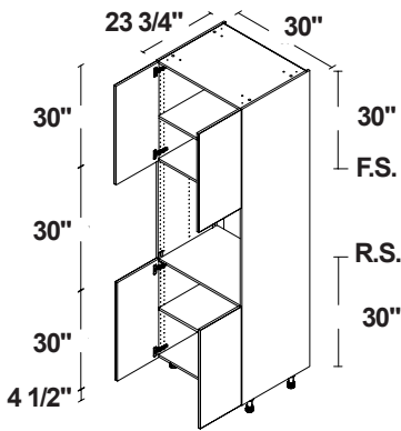
HORNO SIMPLE 3 4 PUERTAS
