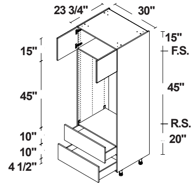
MICRO/HORNO DE PARED 2 2 PUERTAS / 2 CAJONES
