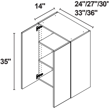
35" DE ALTURA/2 PUERTAS
