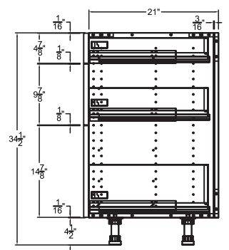
GABINETE DE TOCADOR DE ALTO ESTÁNDAR DE 34 1/2" CON TRES CAJONES
