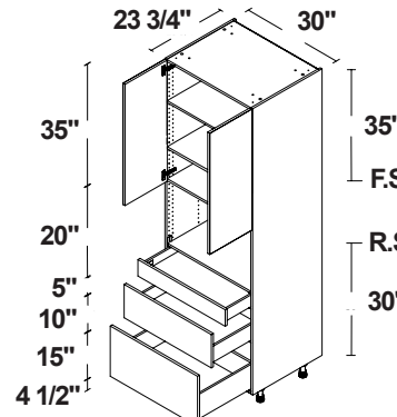
MICROONDAS 1 2 PUERTAS / 3 CAJONES
