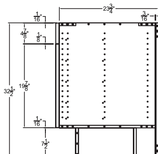
GABINETE BASE ALTO ADA DE 32 1/2"
