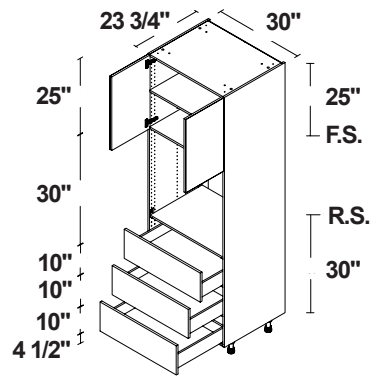
HORNO SIMPLE 3 2 PUERTAS / 3 CAJONES
