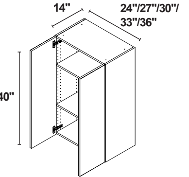
40" DE ALTURA / 2 PUERTAS
