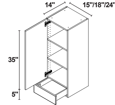
40" DE ALTURA/1 PUERTA / 1 CAJÓN*
