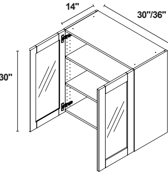
30" DE ALTURA/2 PUERTAS DE VIDRIO*
